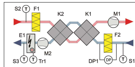
Левостороннее исполнение
